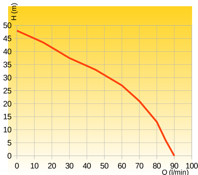
CARATTERISTICA DI FUNZIONAMENTO
